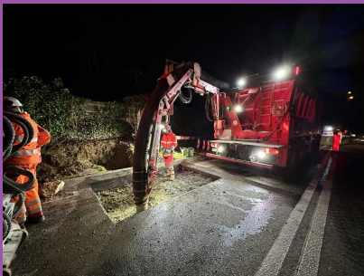
Anschluss Löschwasserprovisorium
